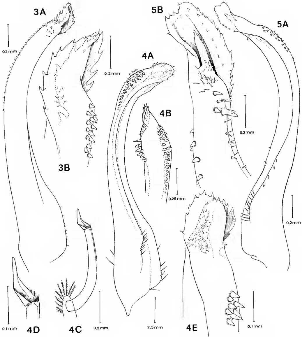
FIG. 3-5. — Pléopodes sexuels mâles dans le genre Garthiope gen. nov. : 3 A, B, G. spinipes (A. Milne Edwards), ♂ 6 × 9 mm, Florida, Tortugas, Bird Key Reef (USNM 75851) : A, P11 en entier ; B, id. , apex. 4 A-D, G. fraseri (Garth), holotype, ♂ 7,4 × 11,1 mm, Galapagos, Charles Island, from Black Beach Anchorage (AHF) : A, P11 en entier ; B, id. , apex ; C, P12 en entier ; D, id. , flagelle ; 4 E, G. fraseri (Garth), paratype, ♂ 6,3 × 9 mm, Galapagos, Barrington Island (MP-B20914) : P11, apex monté en préparation. 5 A, B, G. barbadensis (Rathbun), ♂ 6,8 × 9,5 mm, Florida, Tortugas (ex-USNM 75754 pt. MP-B20916) : A, P11 en entier ; B, id. , apex. (Fig. 4 A-D d'après des dessins originaux de J. S. GARTH et non publiés.)
